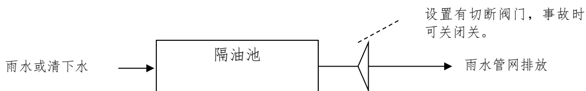
图 1 加油站排水流程示意图
