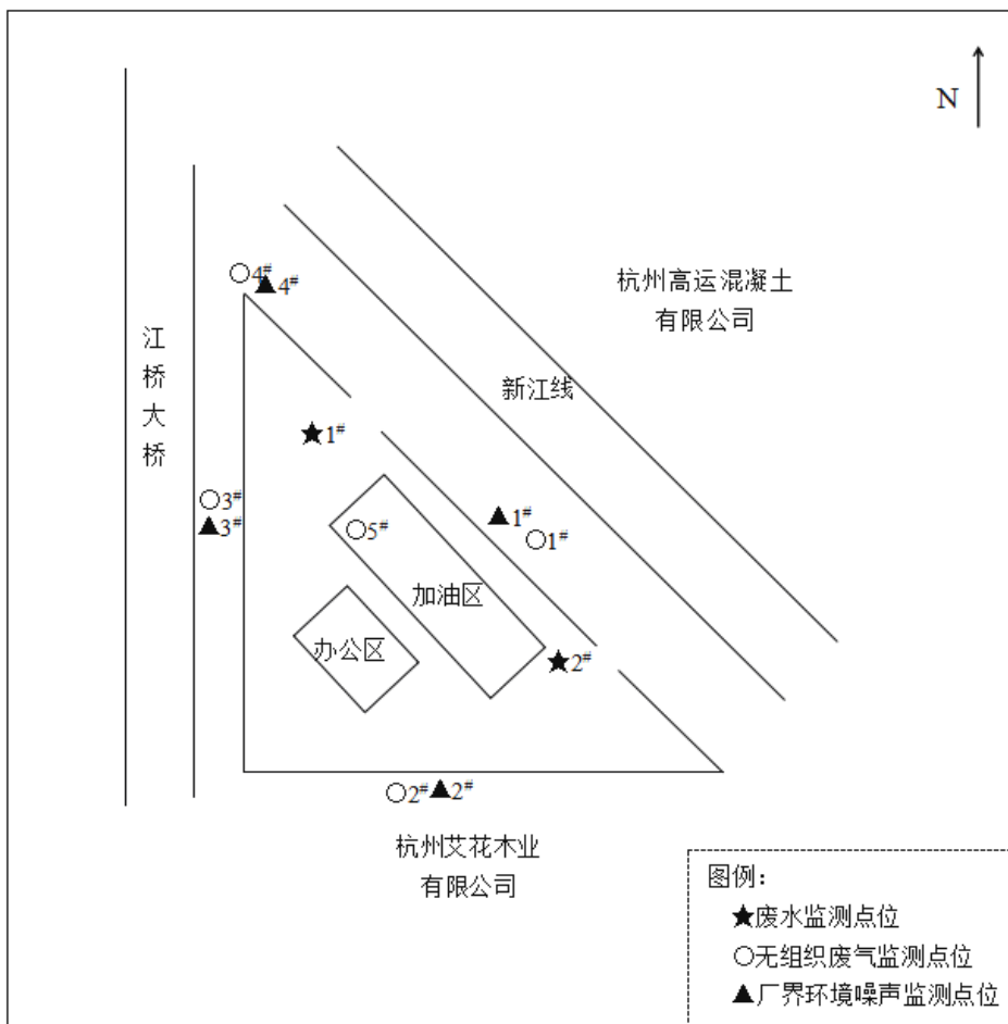
图 3-2 厂区平面布置图及监测点位图
