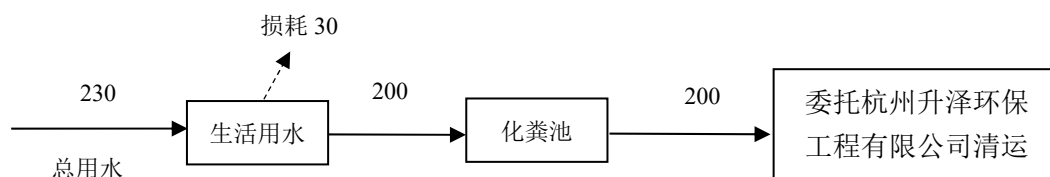
图 3-3 加油站水平衡 单位：t/a
