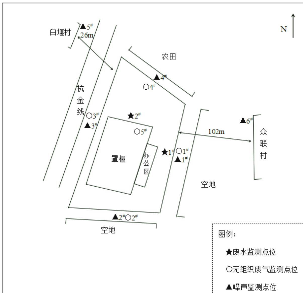
图 3-2 厂区平面布置图及监测点位图
