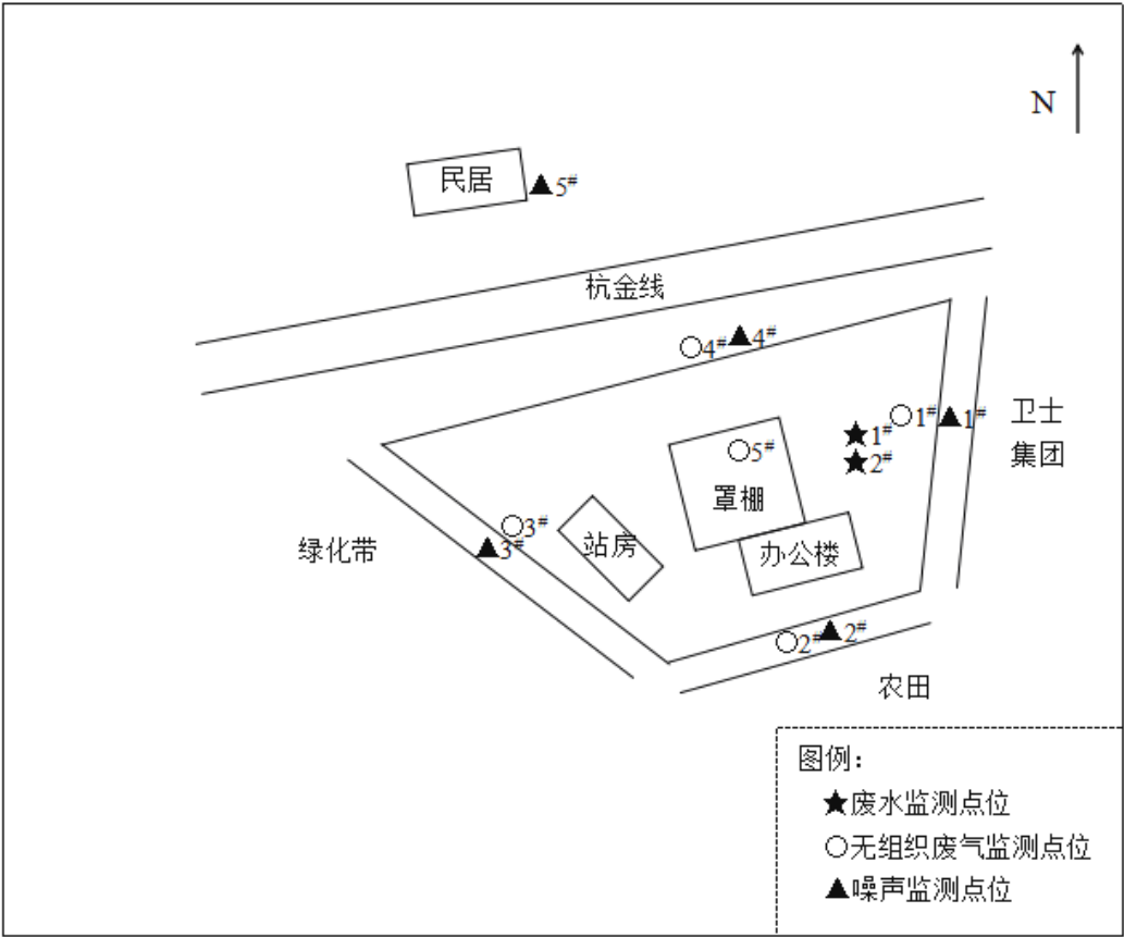
图 3-2 厂区平面布置图及监测点位图
