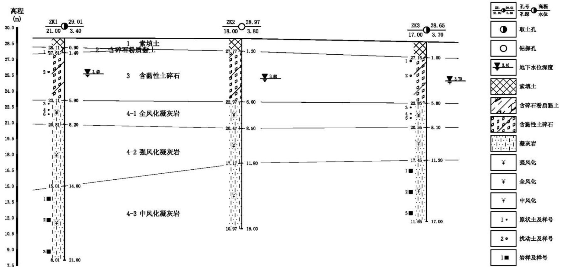
图 3.1-8 工程地质剖面图（部分）
