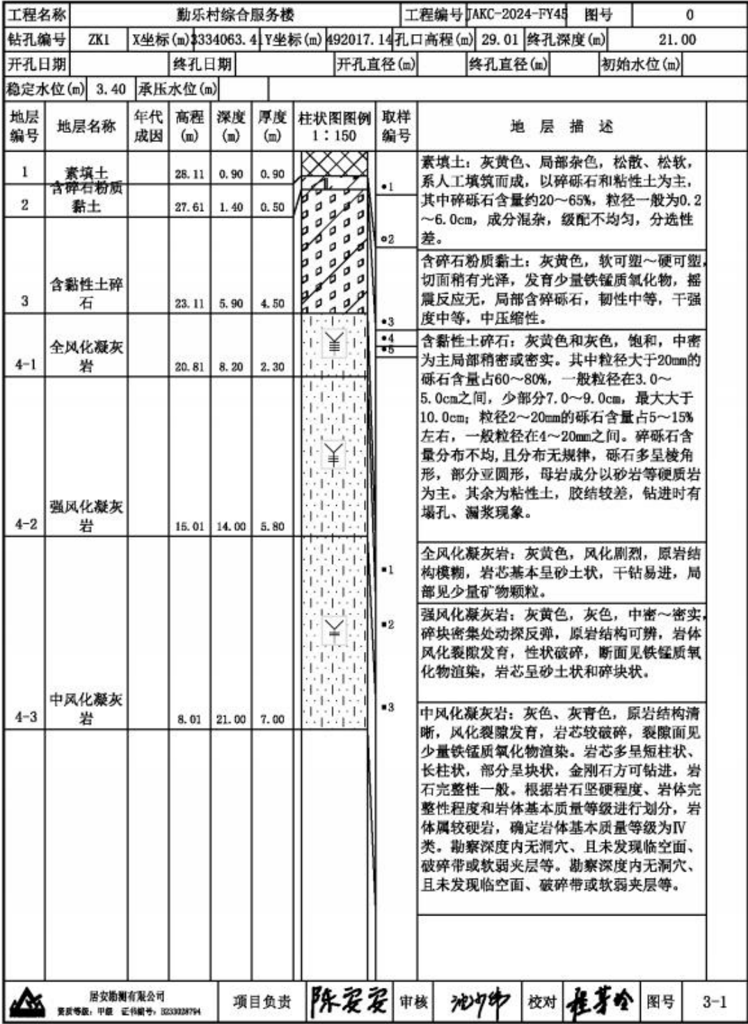
图 3.1-9 地勘钻孔柱状图（部分）
