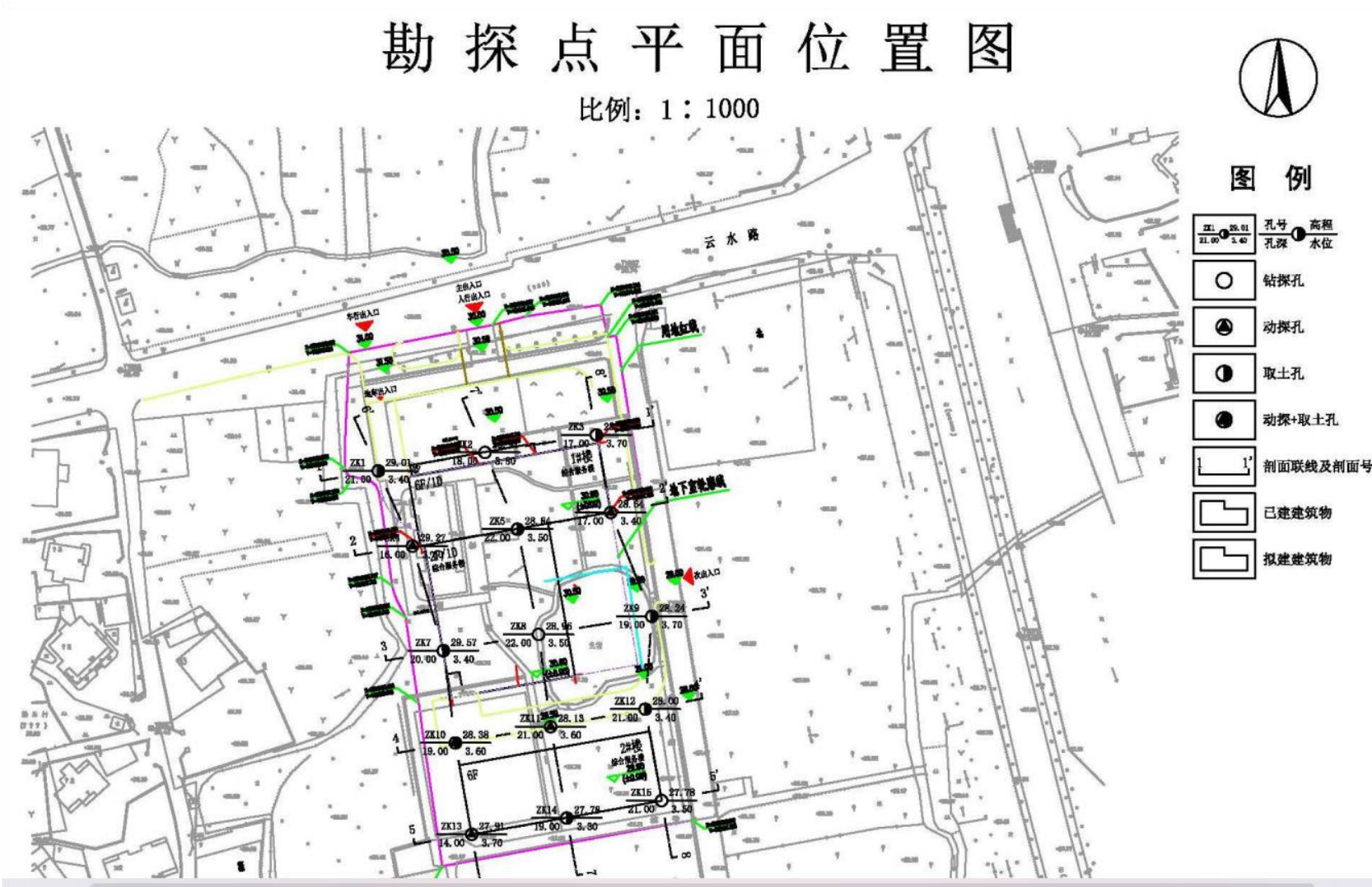
图 3.1-7 勘察点平面位置图
