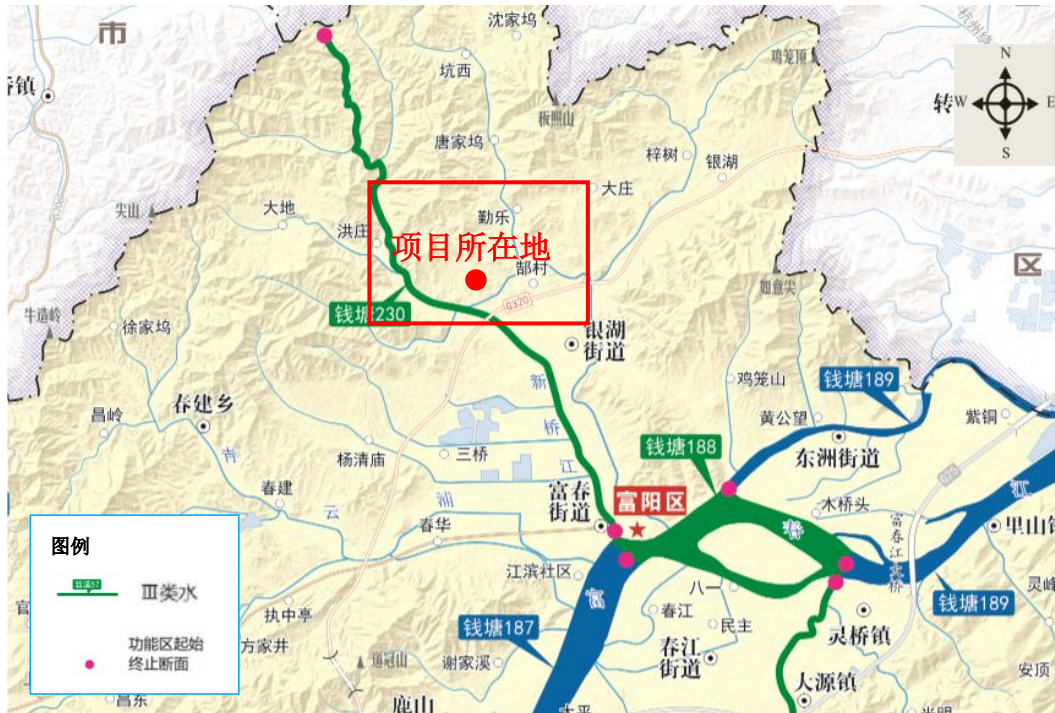
图 3.1-4 调查地块所在区域水环境功能区划图（红色框线标识区域）
