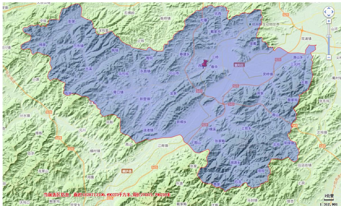
图 3.1-2 富阳区地貌图
